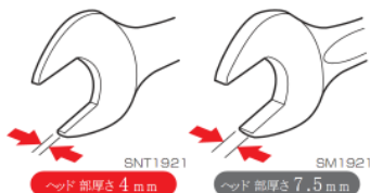
SNT 極薄スパナ
